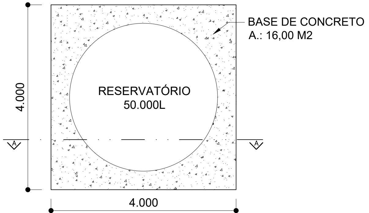
PLANTA BAIXA
