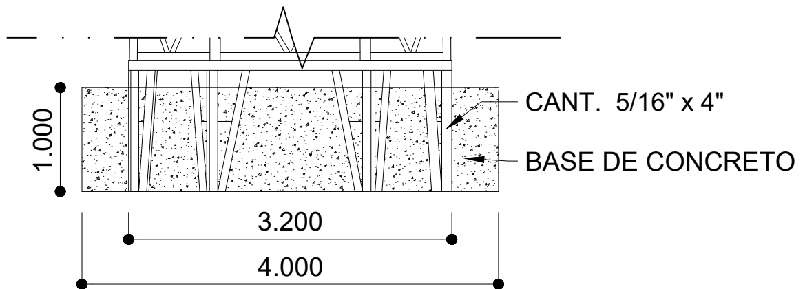
CORTE A-A
