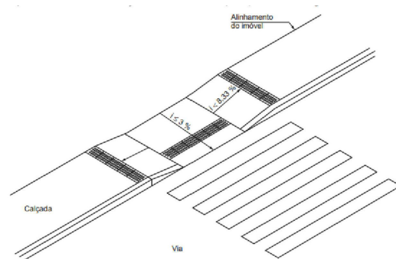
DETALHAMENTO DA RAMPA CONFORME NBR 9050
