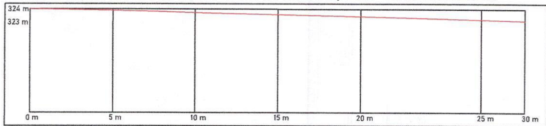
PERFIL LONGITUDINAL: Rodovia RS-155, sentido R. Francisco Sperotto - Acesso bairro Modelo
