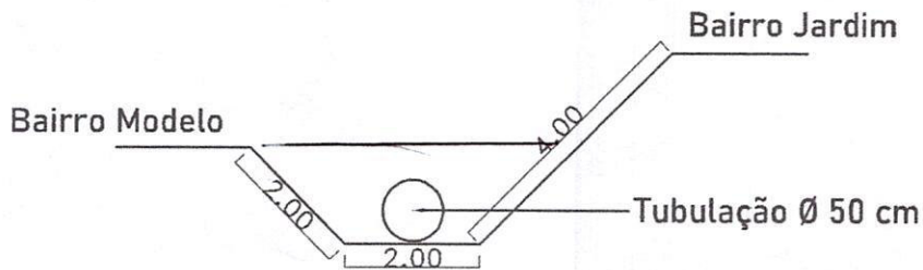
Corte esquemático
