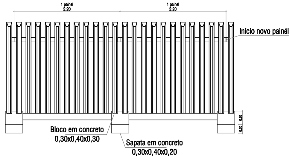
LOCAÇÃO PAINEL DE GRADIL
