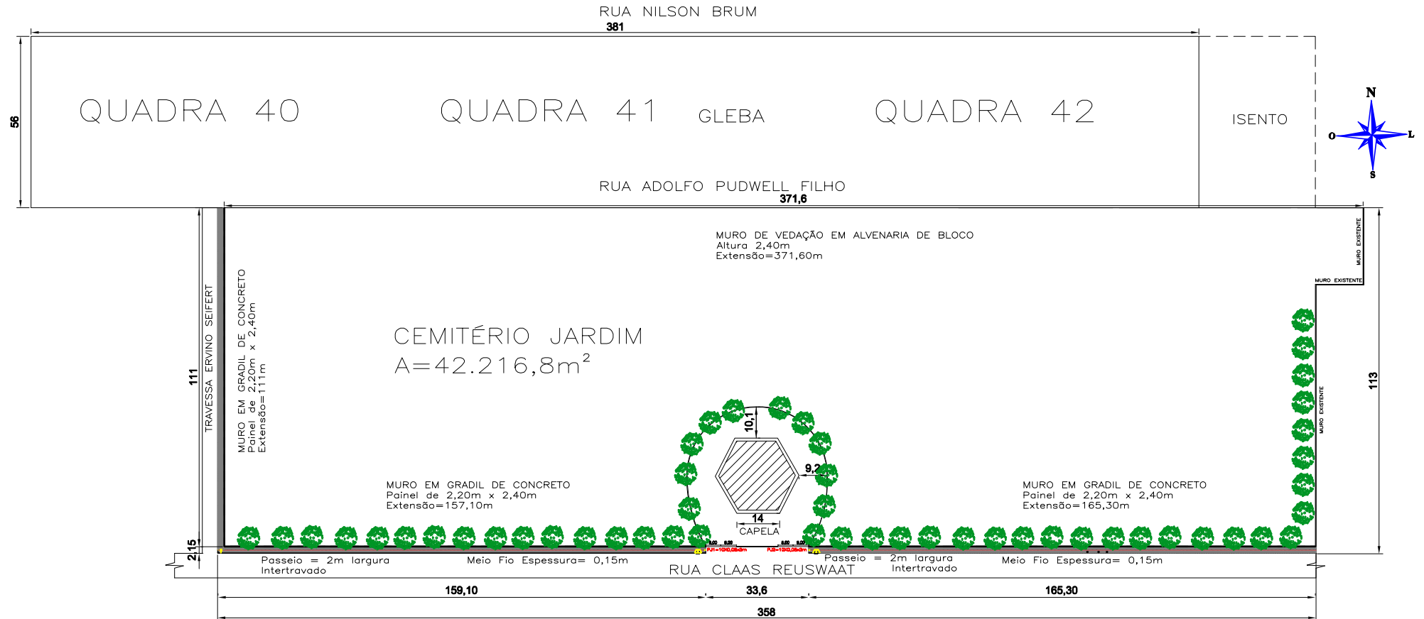
PLANTA BAIXA CEMITÉRIO JARDIM ESC: 1:2
