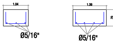
DETALHAMENTO SAPATA
