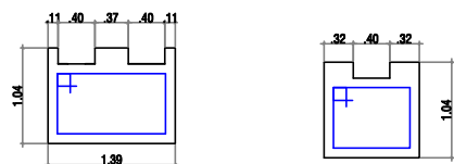
DETALHAMENTO BLOCOS
