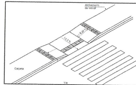
DETALHAMENTO DA RAMPA CONFORME NBR 9050
