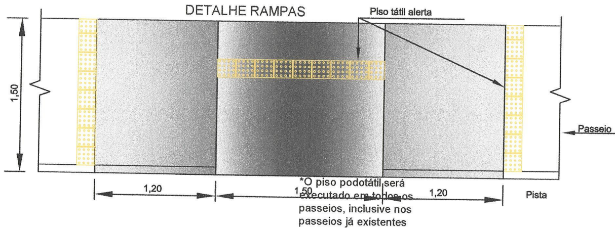
DETALHAMENTO DA RAMPA CONFORME NBR 9050
