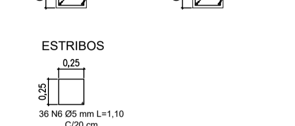
SEÇÃO VIGA AA
