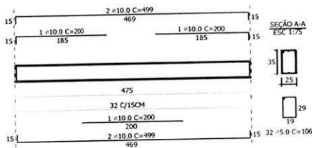
V1 A V3 (3X) 1:50
