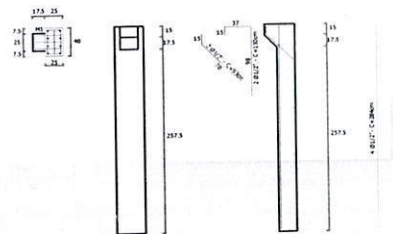
P5 E P8 (2X) 25X40CM 1:50
