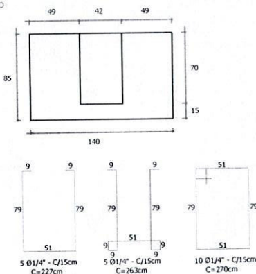
DETALHE BLOCOS DE FUNDAÇÃO ESCALA 1:25
