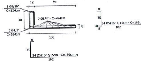
DETALHE POR MÓDULO (3X) DETALHE DEGRAU EM L (1X)
