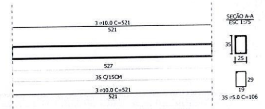
VF7 A VF10 (4X) 1:50
