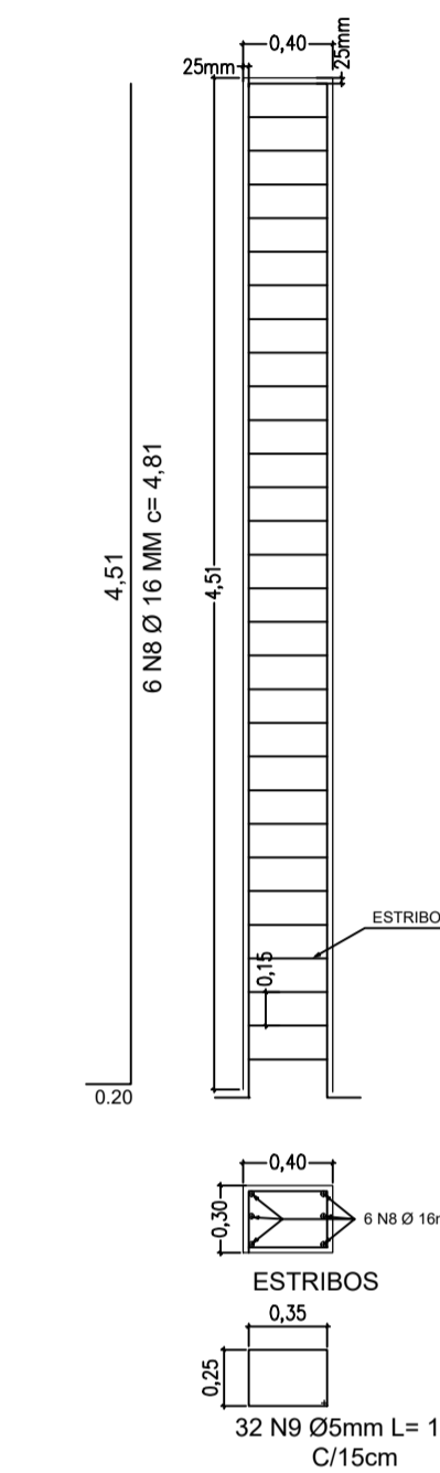
PARTE 1 DETALHAMENTO ARMADURA DOS PILARES P1 = P2 = P3 = P4 = P5 = P6 = P7 - PILARES = 30 x 40 CM
