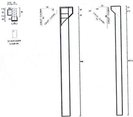
P1 E P4 (2X) 25X40CM 1:50
