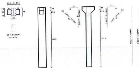
P6 E P7 (2X) 25X40CM 1:50
