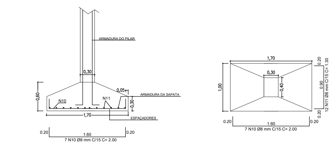
PARTE 1 DETALHAMENTO ARMADURA DAS SAPATAS S1 = S2 = S3 = S4 = S5 = S6 = S7 SAPATAS = (1,70x1,00x0,60 cm)
