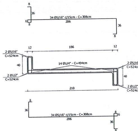
DETALHE POR MÓDULO (3X) DETALHE DEGRAU EM L (1X)
