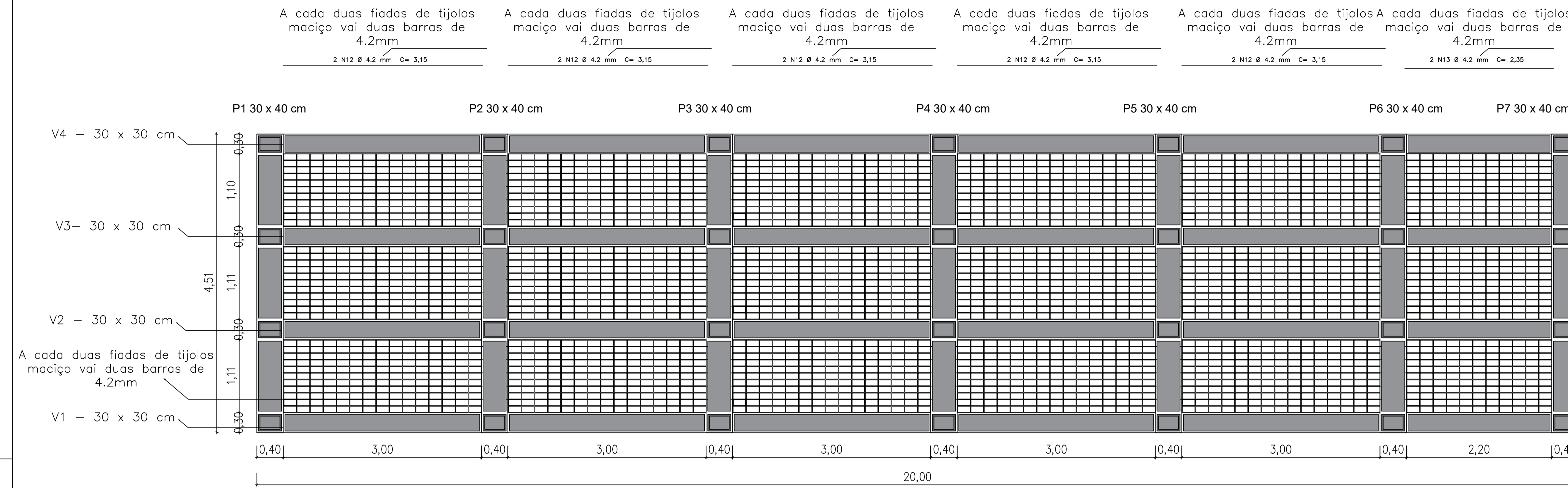
PARTE 1 - DETALHAMENTO ARMADURA DAS V1 - VIGA BALDRAME V2 - VIGA INTERMEDIÁRIA, V3 - INTERMEDIÁRIA E V4- VIGA DE CINTAMENTO
