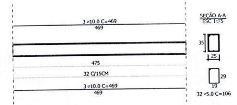
VF1 A VF6 (6X) 1:50
