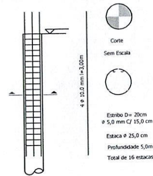
DETALHE DA ESTACA Ø 25 cm ARMADURA DE FUSTE
