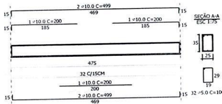
V4 A V6 (3X) 1:50
