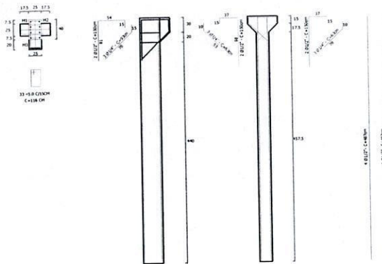
P2 E P3 (2X) 25X40CM 1:50
