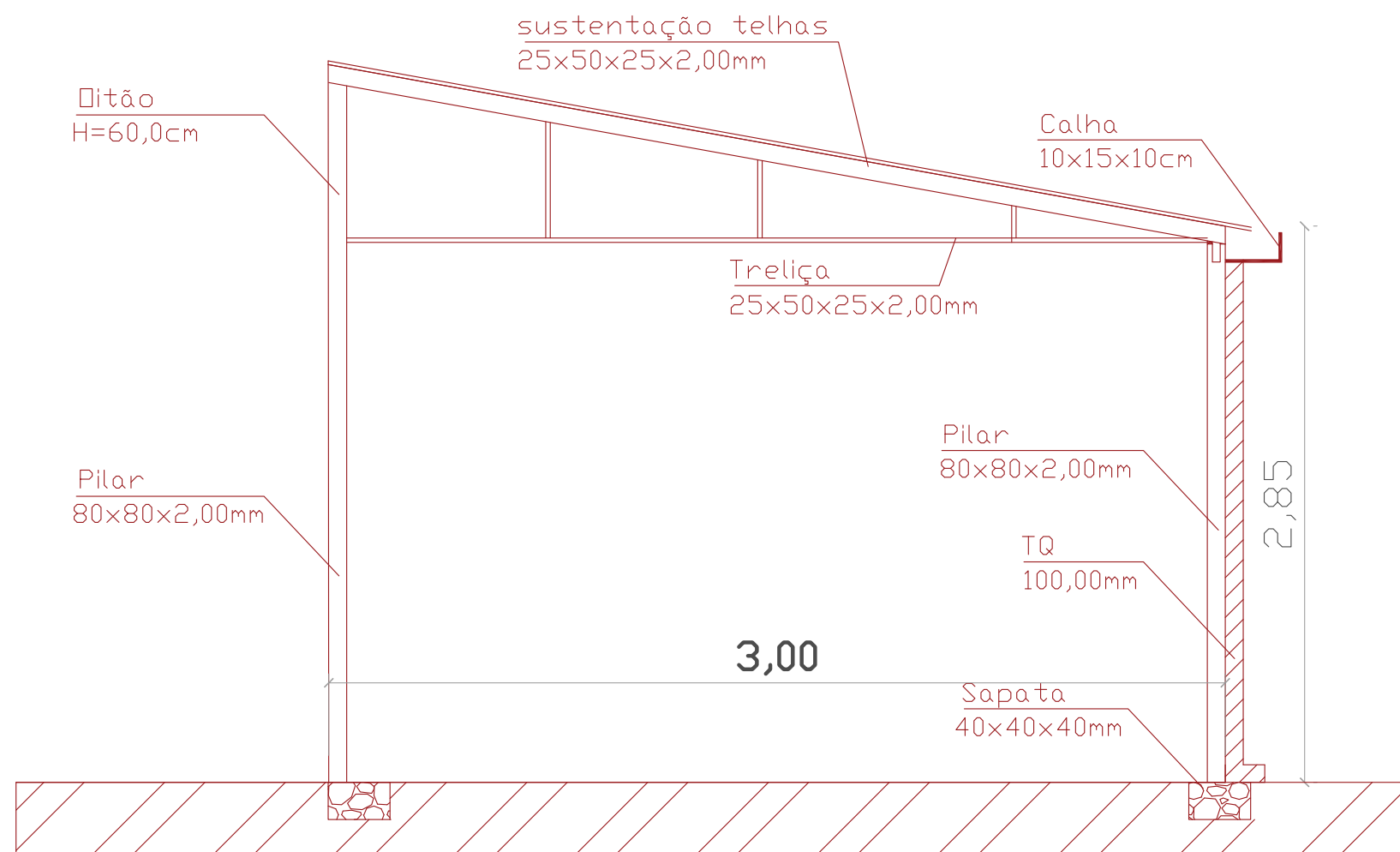
CORTE - Telhado Escala: 1/50
