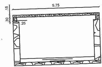
Corte BB
