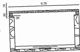
Corte BB
