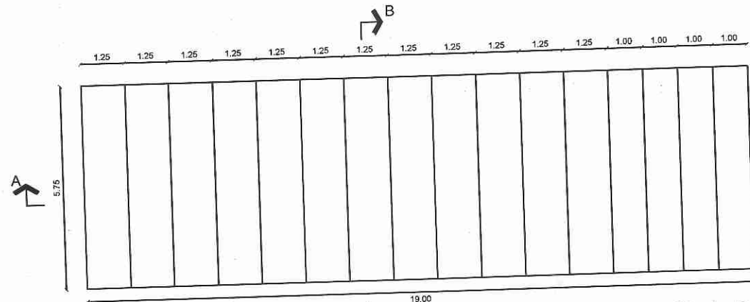
Planta Baixa
