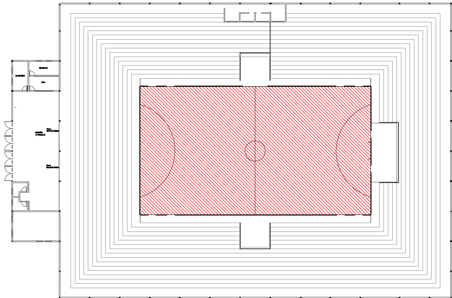
1 PLANTA BAIXA Escala 1:150
